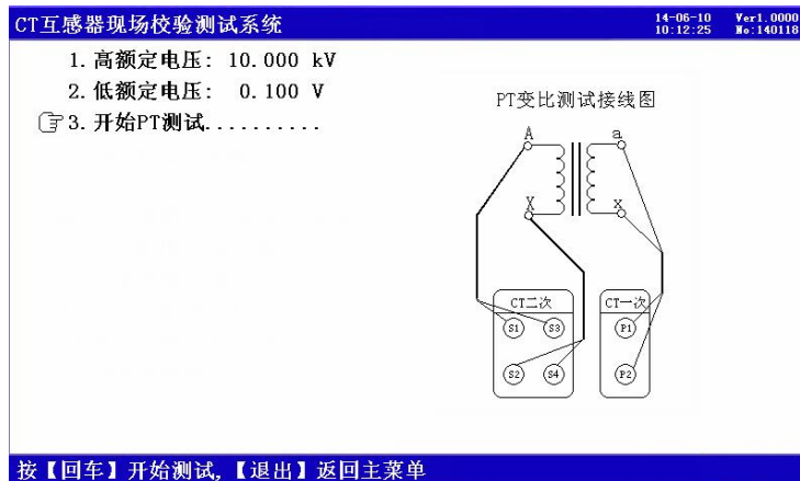
图 12、PT 变比极性设置接线提示界面
