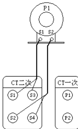
图 17、CT 直阻测试接线示意图
