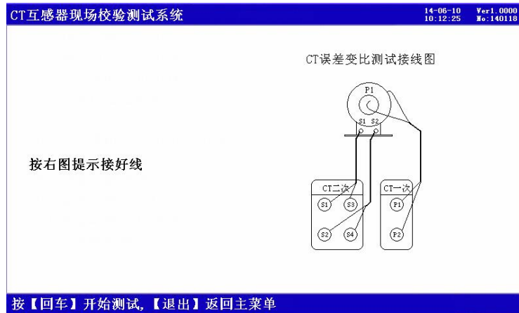
图 10、CT 变比粗测接线提示界面
