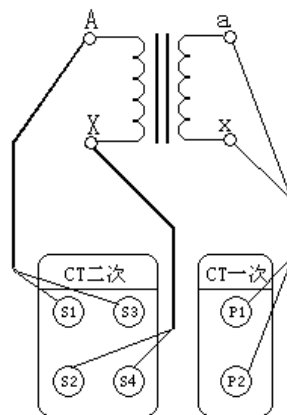
PT变比测试接线图
