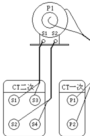
图 16、CT 校验接线示意图
