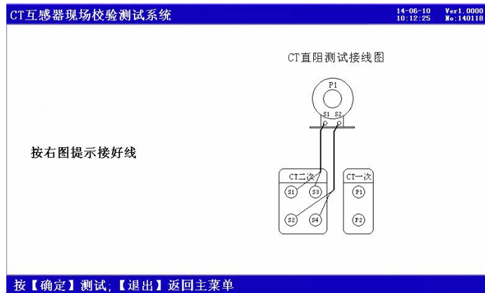
图 8、CT 直阻测试接线提示界面
