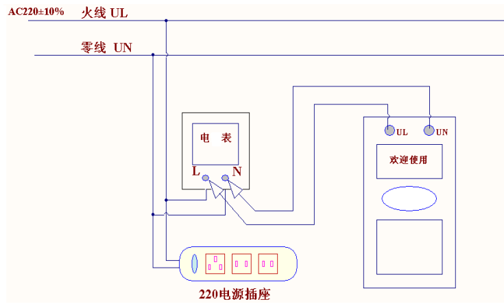
图 11 分机现场接线示意图
