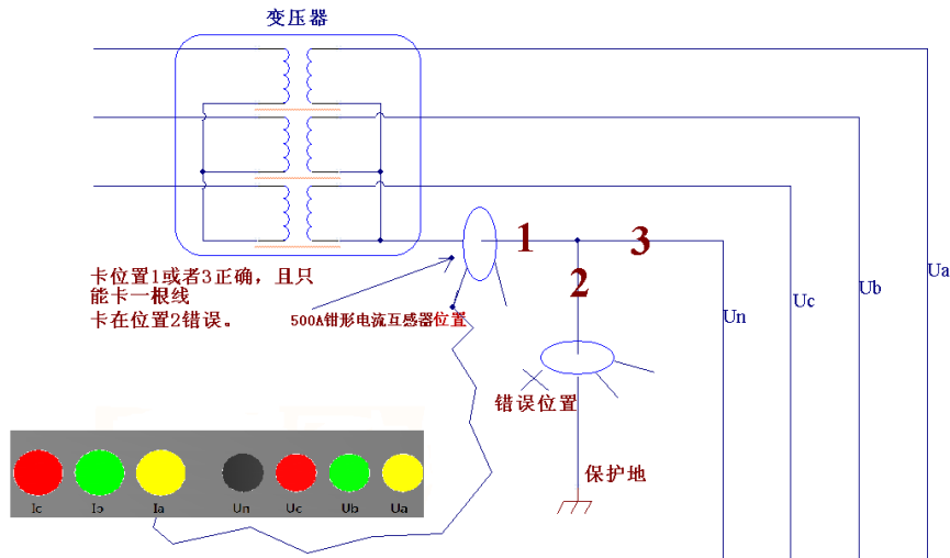
图 5 分支零线钳表正确装钳示意图
