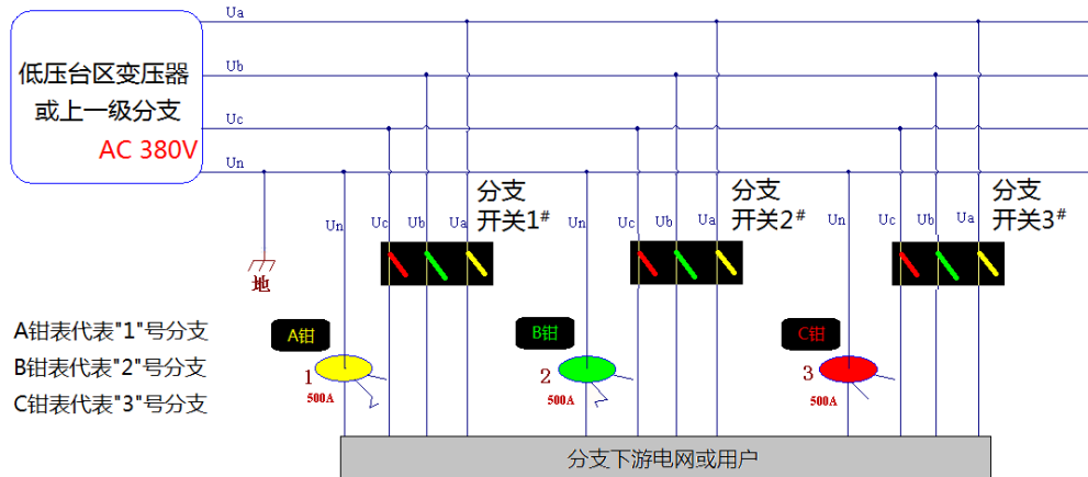
图 2 使用 500A 钳表进行分支测试示意图
